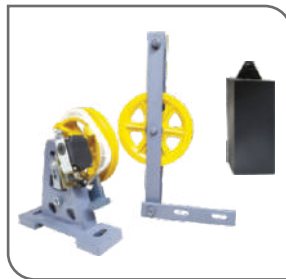
OSG (DIA 200mm)
